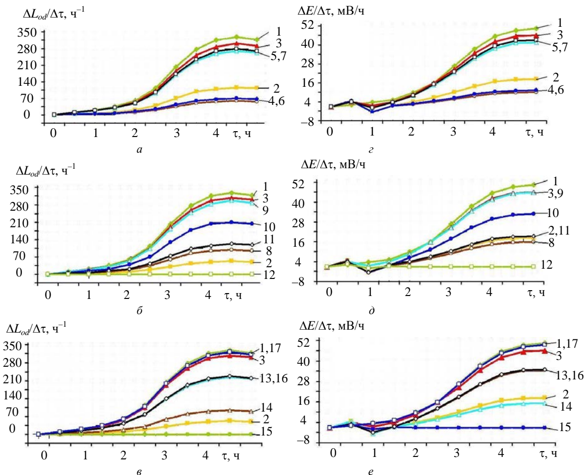
Рис. 3. Усредненные зависимости скоростей изменения эффективности упругого светорассеяния (а–в) и редокс-потенциала (з–е) от времени инкубации E. coli ATCC 25922 в присутствии различных количеств ионов переходных металлов: для контрольных образцов (1), а также для E. coli в присутствии 0,03 М Fe 3+ (2), 0,01 М Fe 3+ (3), 0,03 М Mn 2+ (4), 0,01 М Mn 2+ (5), 0,03 М Cr 3+ (6), 0,01 М Cr 3+ (7), 0,03 М Co 2+ (8), 0,01 М Co 2+ (9), 0,005 М Ni 2+ (10), 0,001 М Ni 2+ (11), 0,0005 М Ni 2+ (12), 0,001 М Cu 2+ (13), 0,0005 М Cu 2+ (14), 0,0002 М Cu 2+ (15), 0,03 М Zn 2+ (16) и 0,01 М Zn 2+ (17)
