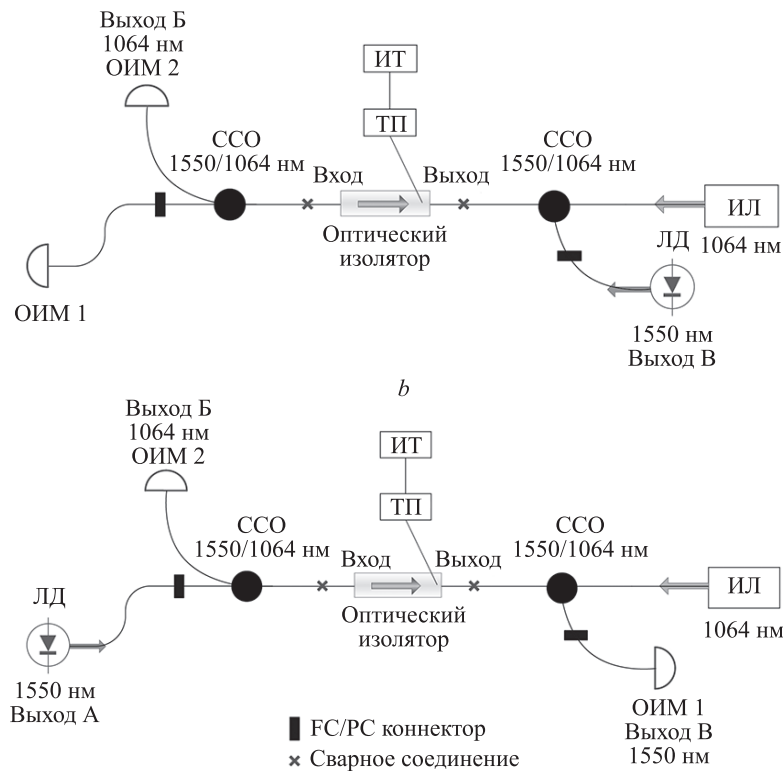
Рис. 2. Схема экспериментальной установки измерения коэффициентов изоляции (а) и вносимых потерь (б). ОИМ 1, 2 — оптический измеритель мощности; ССО — спектрально-селективный ответвитель; ТП — термопара; ИТ — измеритель температуры; ИЛ — импульсный лазер; ЛД — лазерный диод. Стрелки на схеме показывают направление излучения от импульсного лазера и лазерного диода в каждом эксперименте
