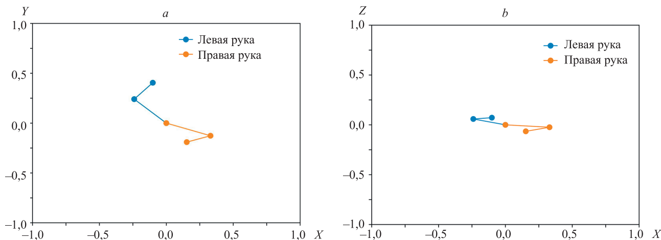
Рис. 2. Результаты работы предложенного метода — проекции расчетного расположения рук в пространстве: плоскостей OXY (a) и OXZ (b). Значения координат нормированы к величине половины диагонали кадра (в пикселях) Fig. 2. Output results of the developed method — projections of estimated spatial arm directions: OXY plane (a) and OXZ plane (b)
