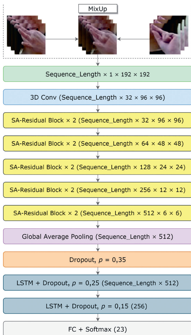
Рис. 3. Архитектура нейросетевой модели E2Ev2 для распознавания конфигураций рук диктора Fig. 3. E2Ev2 architecture of a neural network model for recognizing speaker's hand configurations
