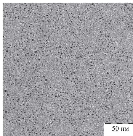
Рис. 1. Изображение наночастиц \text{Ag}_2\text{S} , полученное с помощью просвечивающего электронного микроскопа Fig. 1. Transmission electron microscope image of \text{Ag}_2\text{S} nanoparticles
