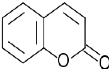
Рисунок 1 – Структурная формула молекулы кумарина Fig. 1 – Structural formula for a molecule of coumarin
