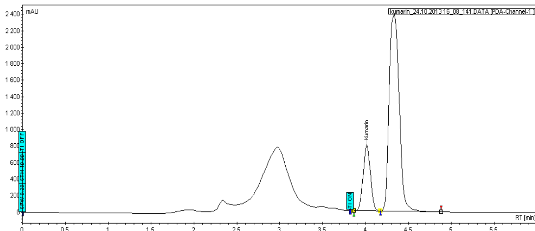
Рисунок 3 – ВЭЖХ-хроматограмма экстракта травы донника, полученного при ультразвуковой экстракции Fig. 3 – High performance liquid chromatography for ularasonic extarction of Melilot's grass
