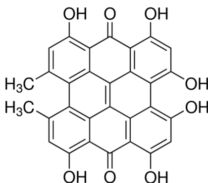
Рисунок 2 – Структурная формула молекулы гиперицина Fig. 2 - Structural formula for a molecule of hypericin
