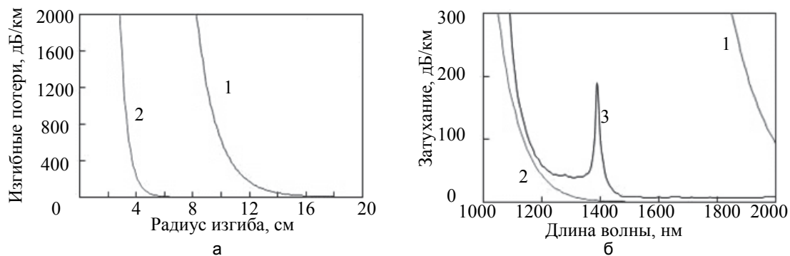
Рис. 4. Изгибные потери на длине волны \lambda = 1550 нм (а) и спектральная характеристика затухания излучения (б) в одномодовом микроструктурированном световоде с сердцевинной диаметром 35 мкм
