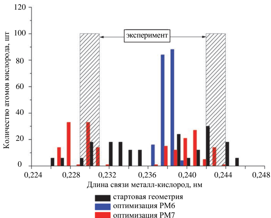
Рис. 3. Гистограмма длин связи Y-O в макроячейке YAG
