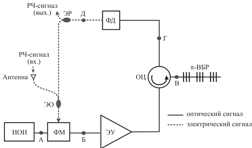
Рис. 7. Детектирование РЧ-сигнала заданной частоты с использованием оптоэлектронного генератора (спектральный РФВОИП № 1), где А, Б, В, Г, Д — участки схемы, на которых необходимо рассмотреть спектры оптического и электрического сигналов
