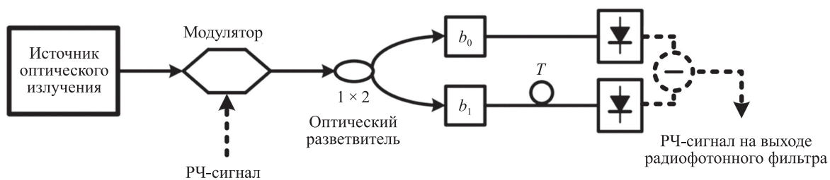
Рис. 3. Структурная схема радиофотонного фильтра с дифференциальным детектированием (радиофотонный фильтр № 2)
