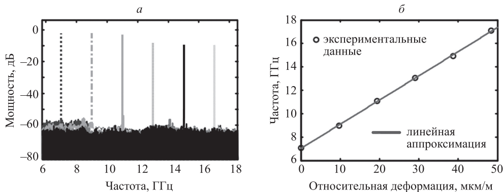
Рис. 10. Частотные спектры оптоэлектронного генератора при разной деформации \pi -ВБР (а); зависимость частоты оптоэлектронного генератора от относительной деформации \pi -ВБР (б)
