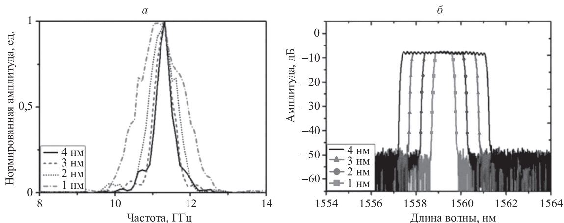
Рис. 15. Амплитудно-частотная характеристика радиопотонного полосового фильтра (а) при различной ширине спектра источника оптического излучения (б)
