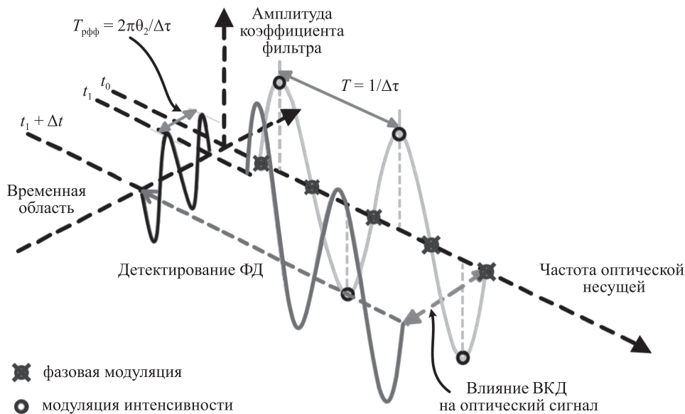
Рис. 14. Схема, поясняющая механизм преобразования оптического сигнала из частотной области во временную: T_{рфф} = 2\pi\theta_2/\Delta\tau — период оптического сигнала во временной области; \theta_2 — общая дисперсия; T — период сигнала в частотной области; t_0 — нулевой момент времени; t_1 — время, которое соответствует появлению оптического сигнала во временной области; \Delta t — длительность оптического сигнала во временной области [26]
