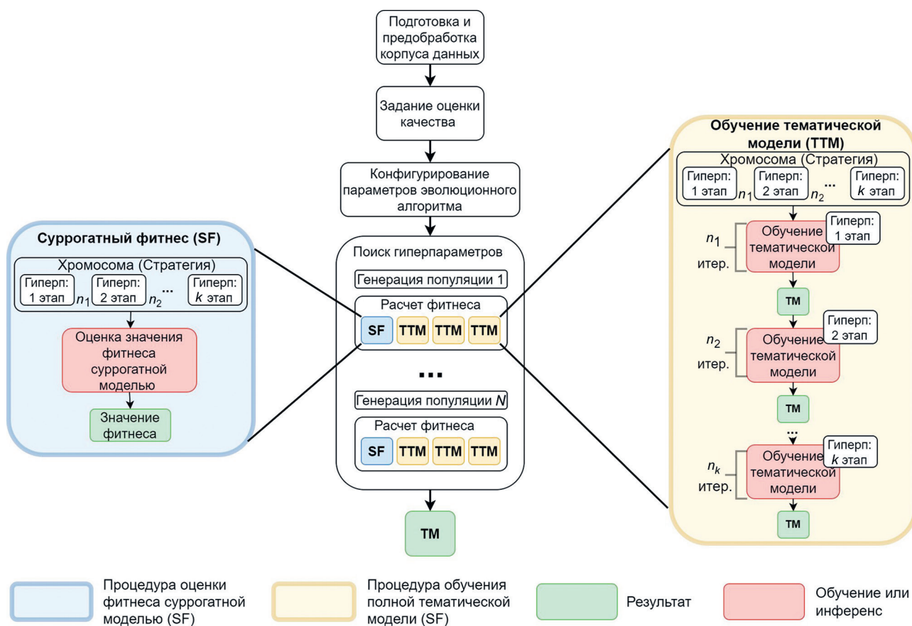
Рис. 2. Общая схема работы фреймворка Fig. 2. The base scheme of the proposed framework
