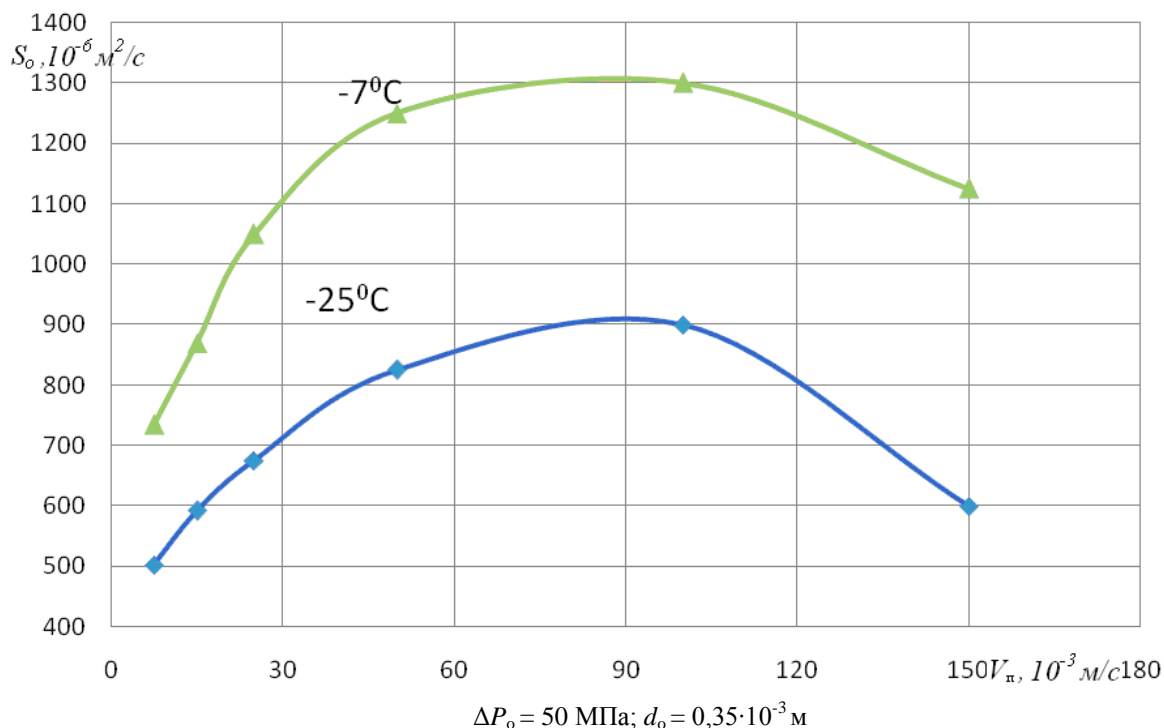
Рисунок 5 – Зависимость скорости приращивания боковой поверхности разреза от скорости перемещения гидроструи относительно разрезаемого образца мяса при l_o = l_{\text{опт}}
