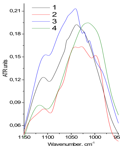
Рисунок 8 – Фрагмент ИК спектров золы образцов корня петрушки: 1 – сырой; 2 – высушен при 50°C; 3 – воздушно-сухой; 4 – лиофилизированный
