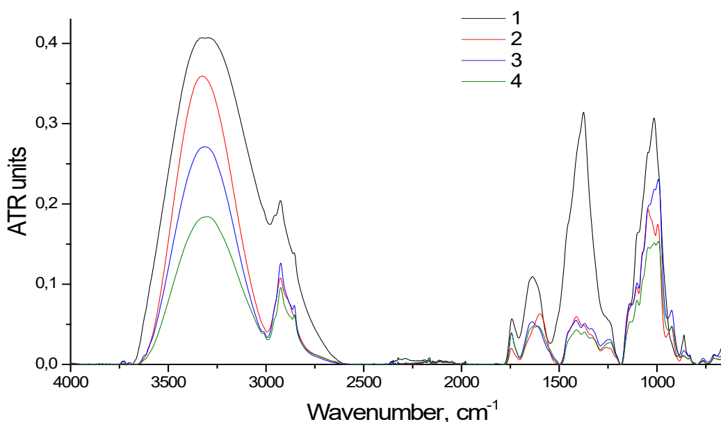
Рисунок 3 – ИК спектры образцов корня петрушки: 1 – сырой; 2 – высушен при 50°C; 3 – воздушно сухой; 4 – лиофилизированный
