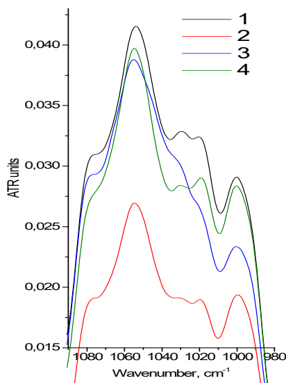
Рисунок 5 – Фрагмент ИК спектров концентратов водных экстрактов корня петрушки в области поглощения углеводных компонентов: 1 – сырой; 2 – высушен при 50°C; 3 – воздушно сухой; 4 – лиофилизированный
