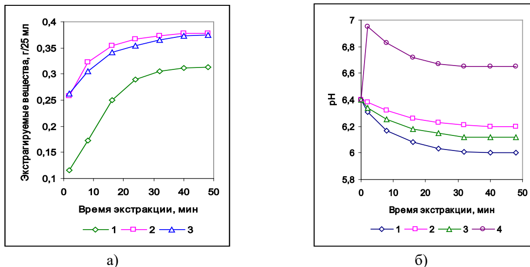
Рисунок 1 – а) Кинетические кривые выхода экстрагируемых веществ; б) Изменения рН в процессе экстракции образцов корня петрушки: 1 – воздушно-сухой; 2 – лиофилизированный; 3 – сушка при 50°C; 4 – сырой
