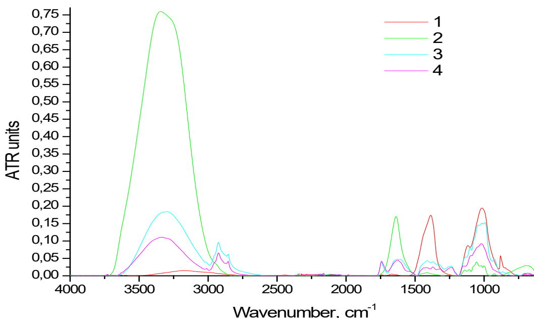
Рисунок 9 – ИК спектры лиофилизованного корня петрушки: 1 – зола; 2 – концентрат водного экстракта; 3 – корень сухой; 4 – воздушно сухой шрот
