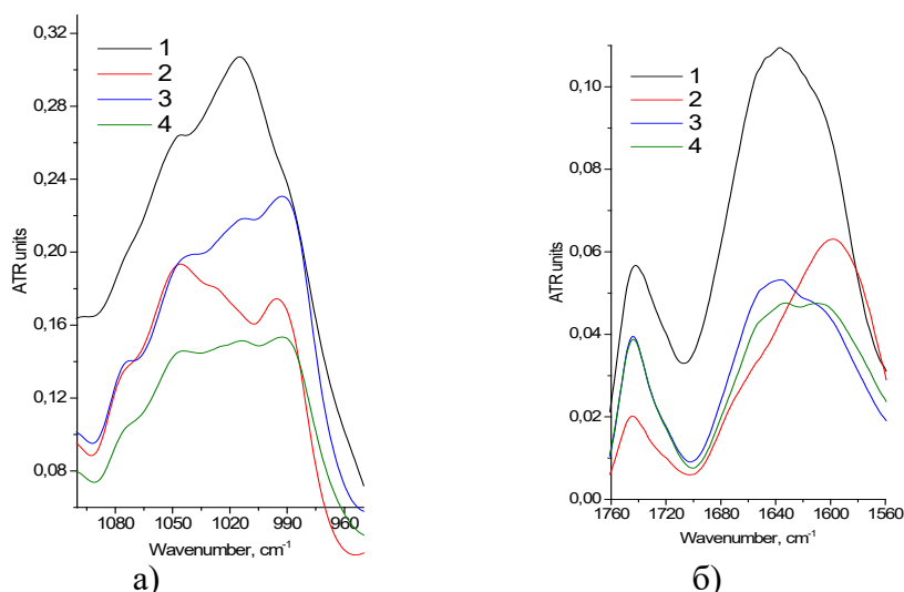
Рисунок 4 – Фрагменты ИК спектров образцов корня петрушки, представленных на рисунке 3: 1 – сырой; 2 – высушен при 50°C; 3 – воздушно сухой; 4 – лиофилизированный
