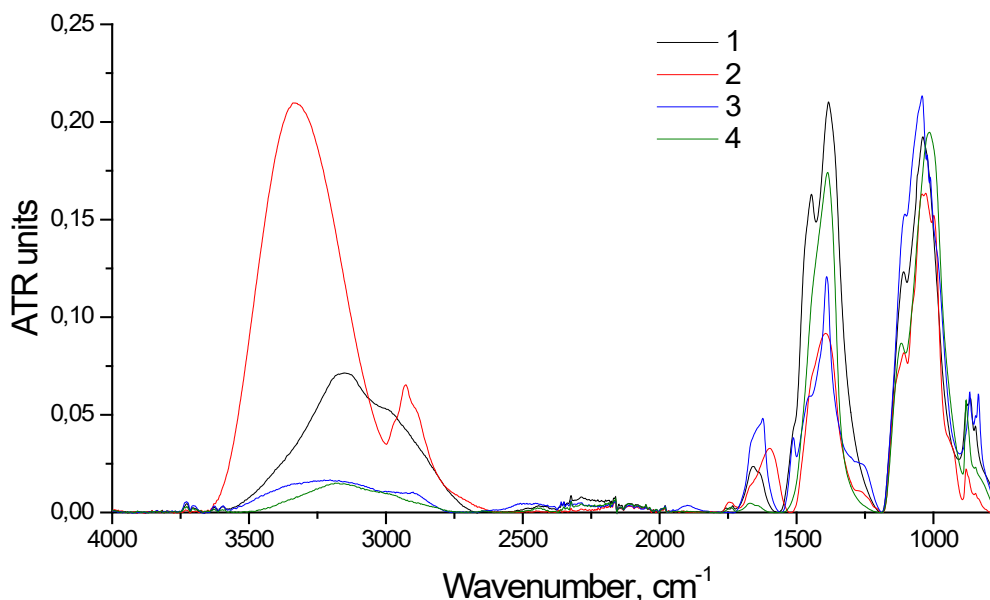
Рисунок 7 – ИК спектры золы образцов корня петрушки: 1 – сырой; 2 – высушен при 50^{\circ}\text{C} ; 3 – воздушно-сухой; 4 – лиофилизованный
