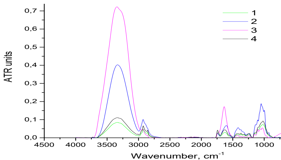
Рисунок 6 – ИК спектры воздушно сухих шротов корня петрушки: 1 – сырой; 2 – высушен при 50°C; 3 – воздушно сухой; 4 – лиофилизированный
